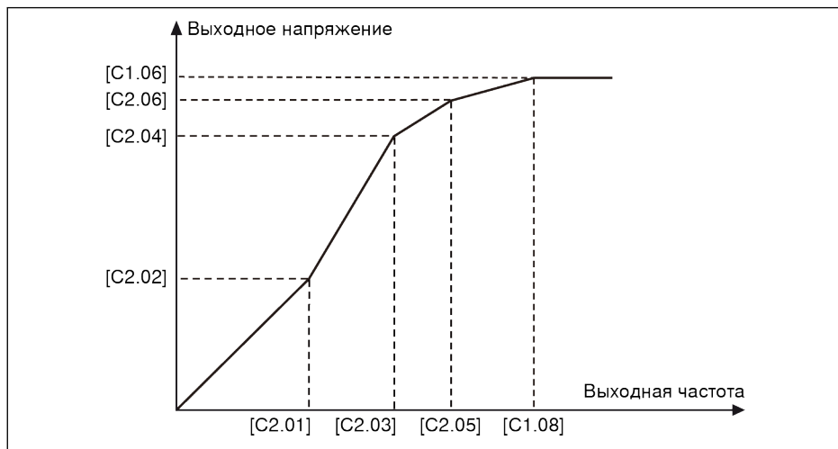
Рис. 12-56: Задаваемая пользователем кривая V/f при [C2.05] \leq [C1.08]
